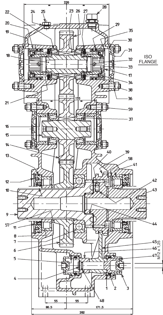
SECTION A-A
