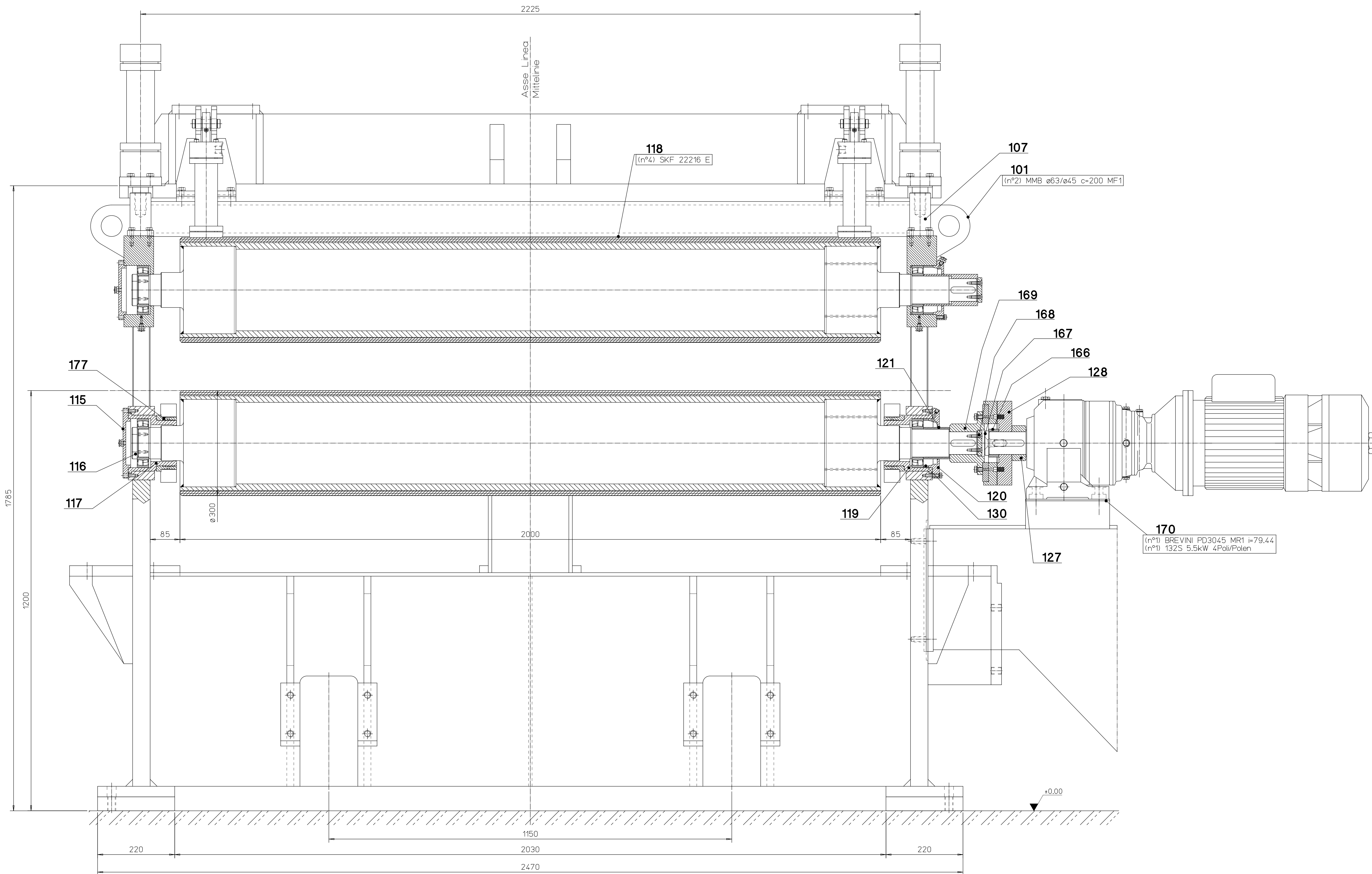
Schnitt Sez. A-A
