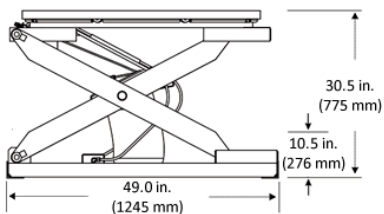
EZ Loader, EZ Loader-E & EZ Loader-SS Specifications
